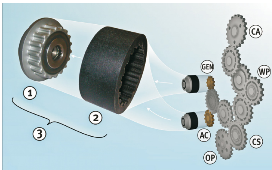
Foto 1: Sprzęgiełko alternatora z elastyczną nasadką w połączeniu czołowym
